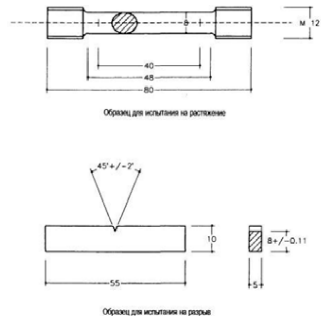
Рисунок А.8. Образцы для испытания на растяжение и на разрыв
