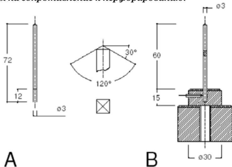
Рисунок А.5. Устройство крепления образцов ткани для испытания одежды на сопротивление к перфорированию
