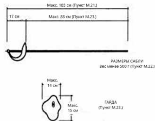
Рисунок 12б. Размеры сабли
