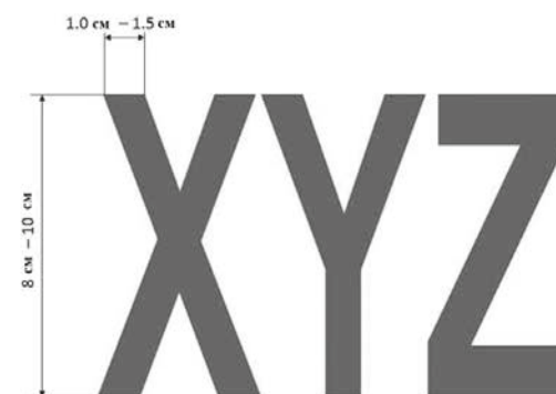
Рисунок 19. Размеры надписи
